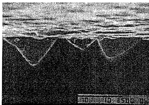
Figura 3.1 Tracce in un SSNTD
