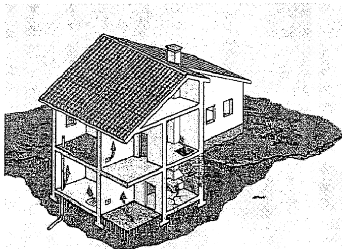
Figura 2.6 Vie d'ingresso del radon in un edificio
