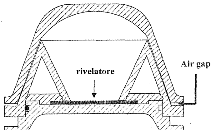
Figura 3.6 Particolare dell'air gap del dosimetro ENEA-IRP in foto e in sezione
