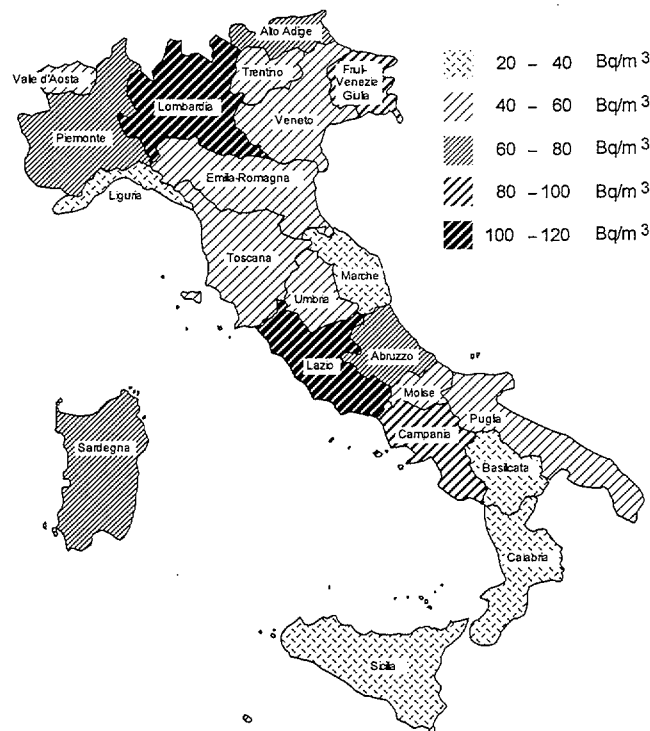
Figura 2.7 Mappa dei valori medi regionali di concentrazione di radon nelle abitazioni italiane, ottenuta nell'ambito dell'Indagine nazionale sulla radioattività naturale nelle abitazioni" (13)
