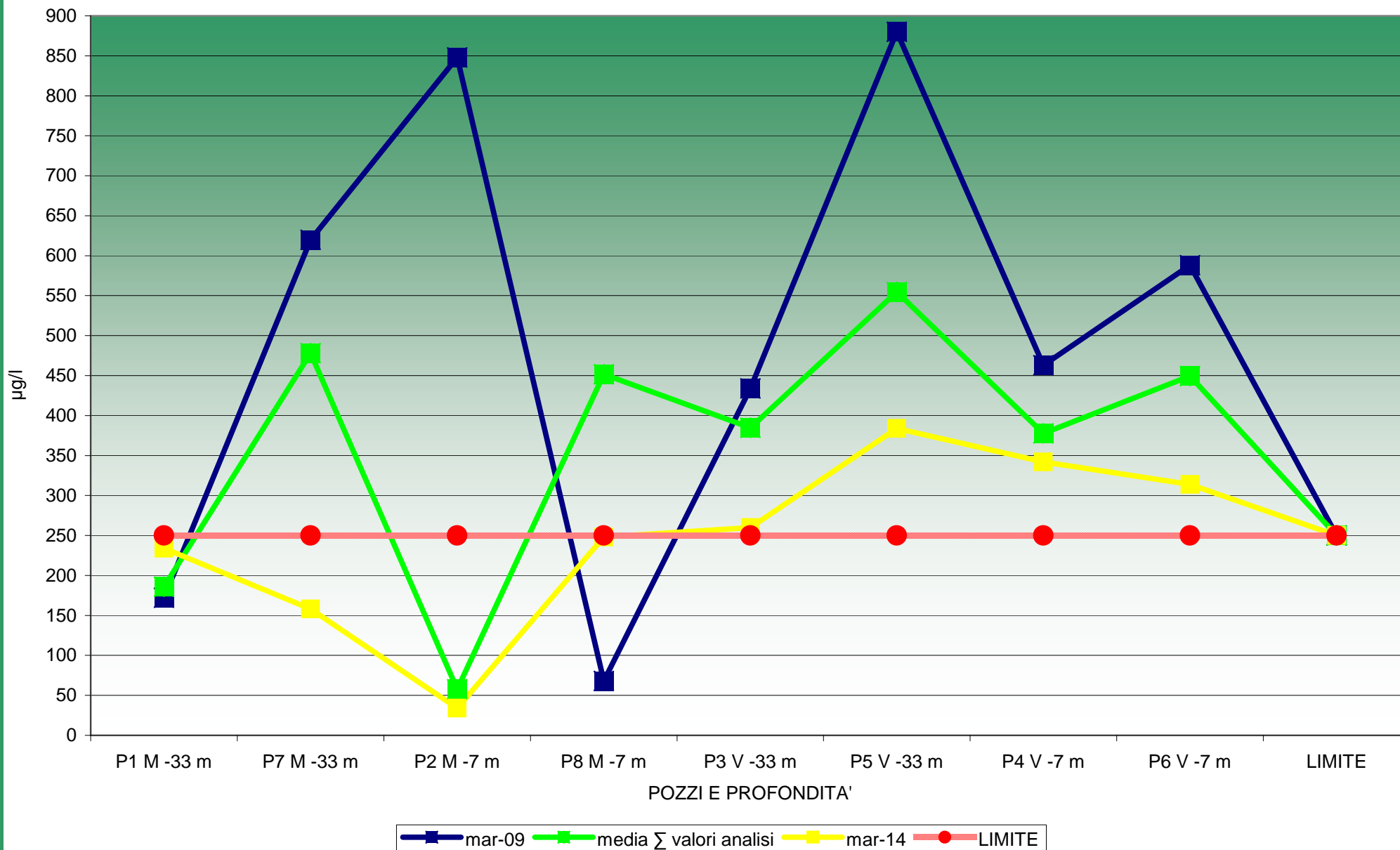
GRAFICO N. 16 INCENERITORE CON RECUPERO DI ENERGIA DI ACERRA (NA) CONFRONTO DI SOLFATI IN FALDE SUPERFICIALI (-7 m) - PROFONDE (-33 m) - MONTE (M) - VALLE (V) TRA BIANCO AMBIENTALE (MARZO-2009) ULTIMA VERIFICA (MARZO-2014) E MEDIA \Sigma VALORI ANALISI
